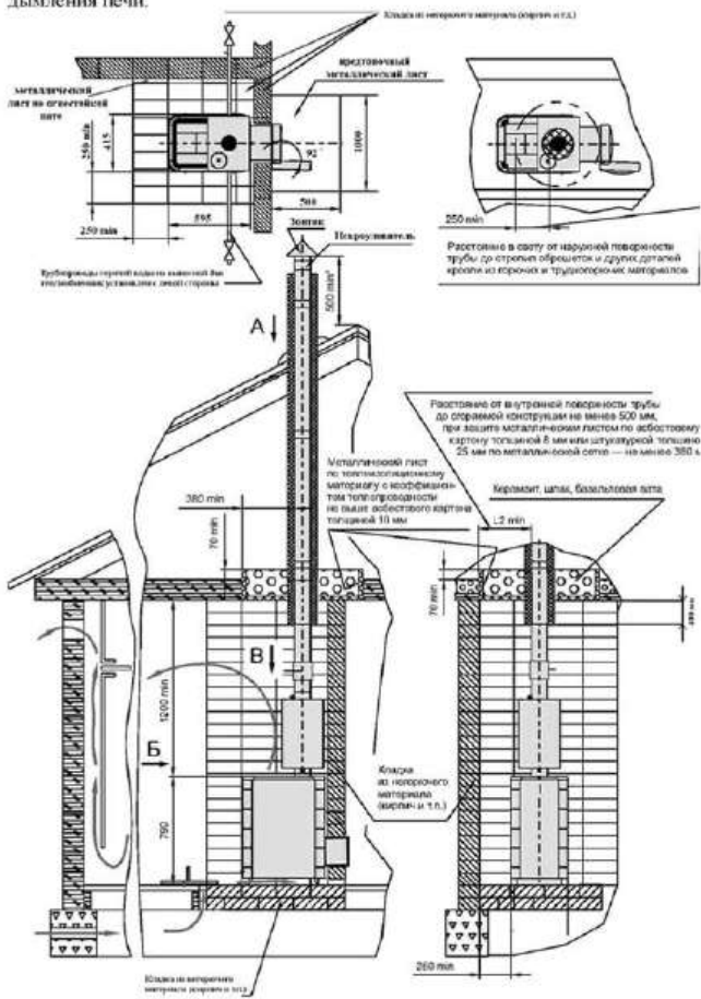
Схема монтажа печи
