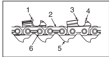
Рис. 27 Конструкция пильной цепи
