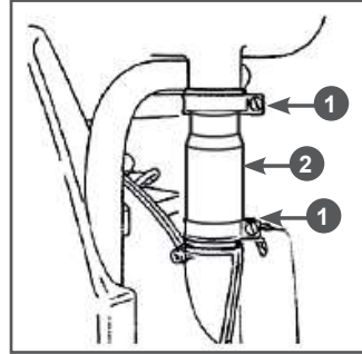
Рис. 14 Снятие впускного шланга распылителя
