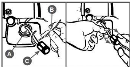
Рис. 22 Извлечение топливного фильтра
