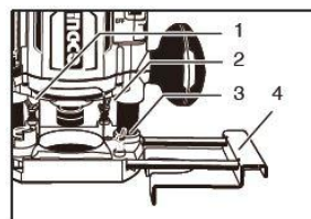
1. Барашковый болт (A) 2. Барашковый болт (B) 3. Барашковый болт (A) 4. Прямая направляющая
