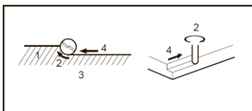
1. Обрабатываемая деталь 2. Направление вращения биты 3. Вид сверху инструмента 4. Направление подачи
