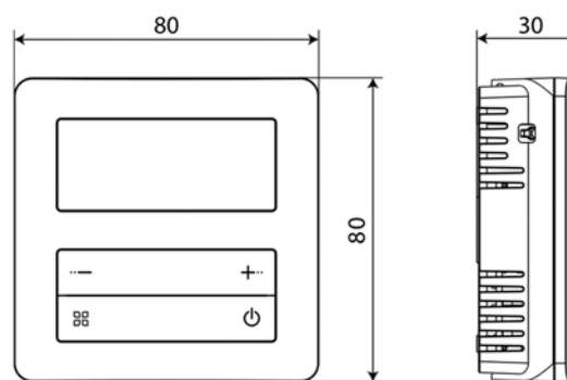
Габаритные размеры терморегулятора, мм
