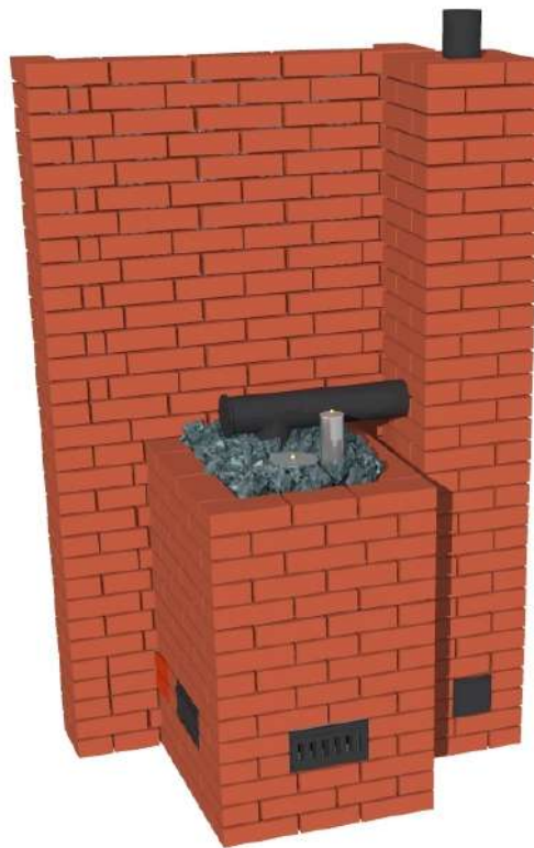
Рис. 11 Пример установки печи в кирпичном кожухе с отдельно стоящим ДЫМОХОДОМ
