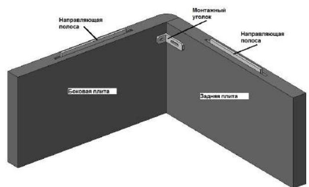
Рис. 6 Расположение монтажного уголка и металлических полос
