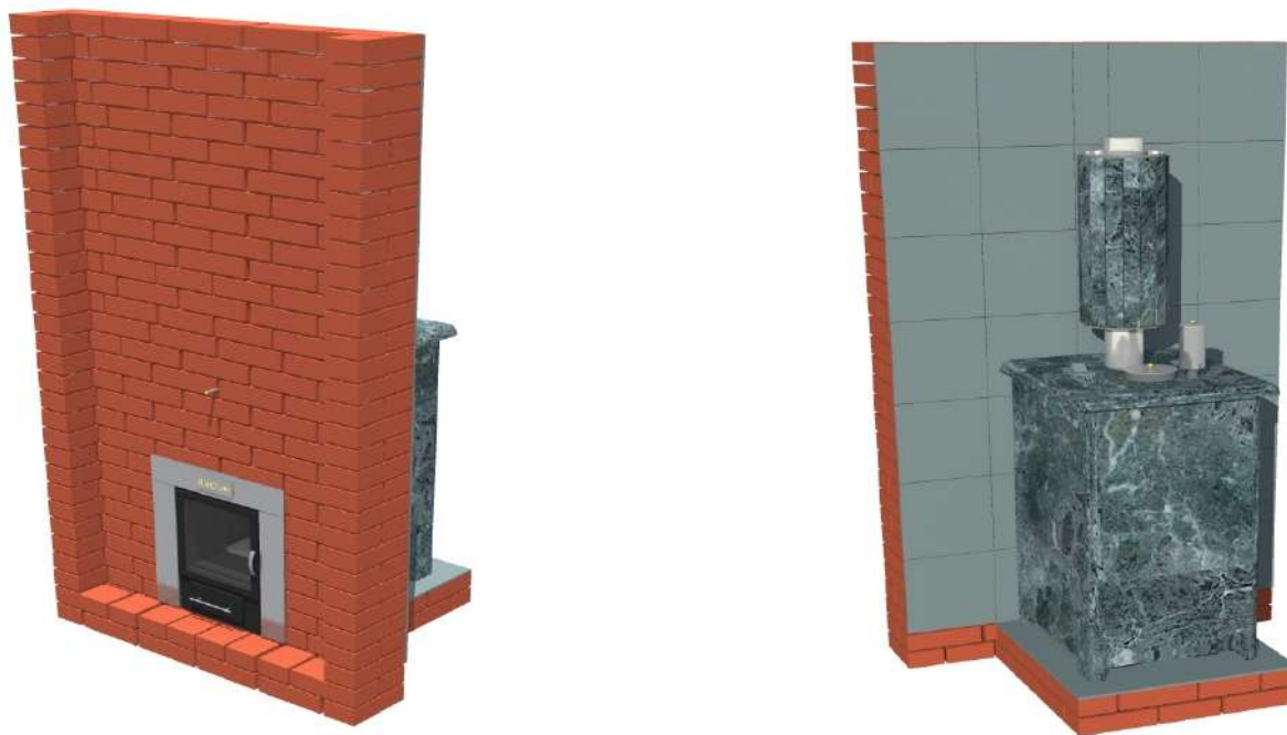
Рис. 4 Пример установки печи в облицовке из природного камня
