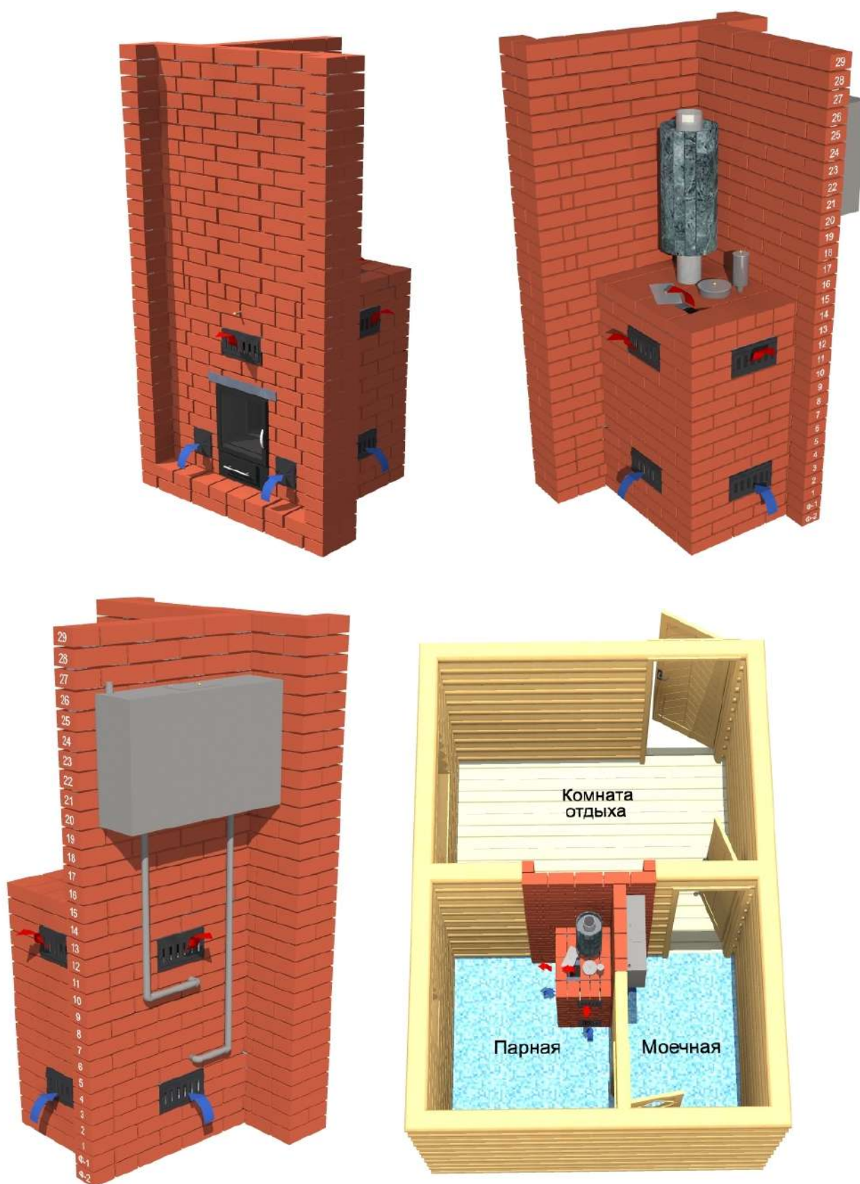
Рис. 8 Пример установки печи в кирпичном кожухе с функцией обогрева комнаты отдыха и моечного отделения
