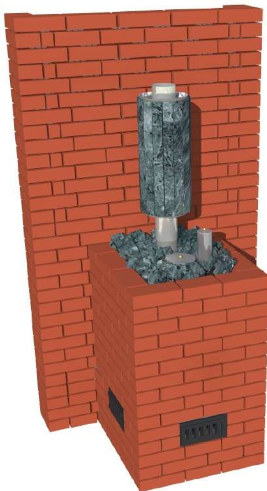
Рис. 9 Пример декорирования верха печи камнями
