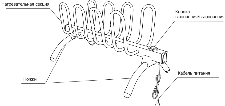
Рисунок 1. Устройство сушилок для обуви
