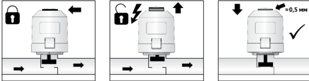
Вид правильно установленного привода
