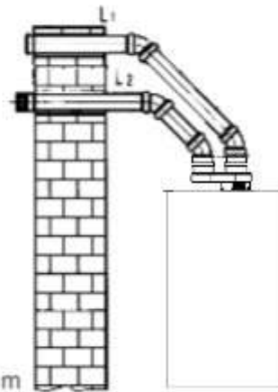
(L1+L2)_{max} = 15 метров
