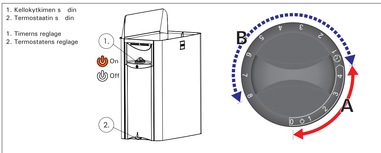
Kuva 2. S-timer (SW45, SW60, SW80, SW90) Bild 2. Reglagen (SW45, SW60, SW80, SW90)
