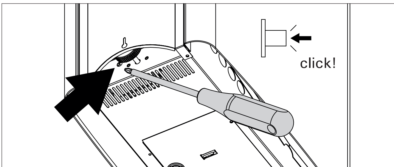
Kuva 12. Ylikuumenemissuojan palautus Bild 12. terst lning av verhetningsskyddet
