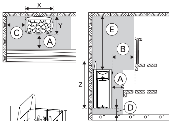
SW45, SW60, SW45E, SW60E : 490 mm SW80, SW90, SW90E: 580 mm
