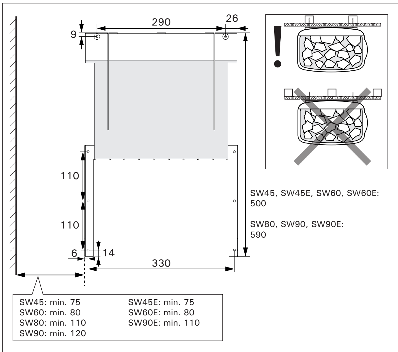
Kuva 7. Sein teline, mitat millimetrein Bild 7. V ggkonsolen, m tten i millimeter
