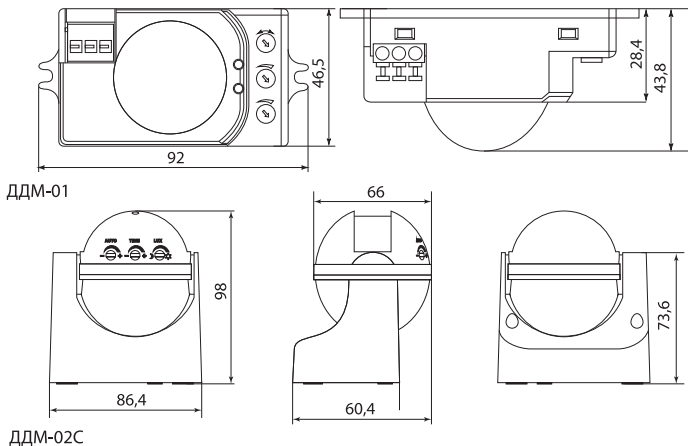
Рисунок 4. Габаритные и установочные размеры датчиков ДДМ-01, ДДМ-02С, мм
