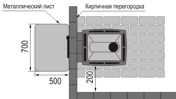
Рисунок 3. Схема установки печи (вид сверху)
