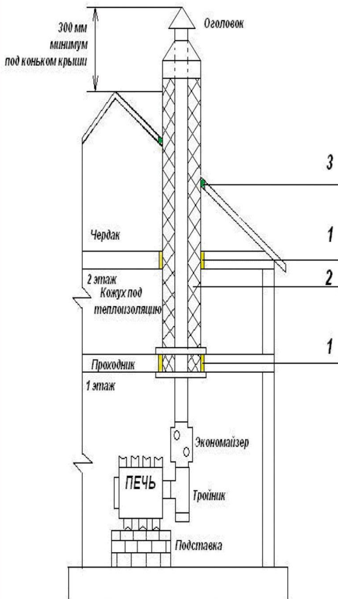
УСТАНОВКА ПЕЧИ С МЕТАЛЛИЧЕСКИМ ДЫМОХОДОМ ВНУТРИ 2-ЭТАЖНОГО ДОМА
