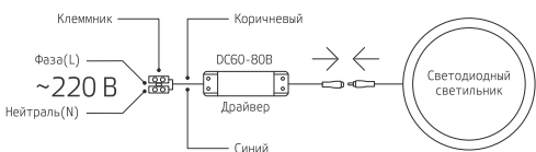
Рис. 2. Схема подключения светодиодного светильника к электросети 220 В
